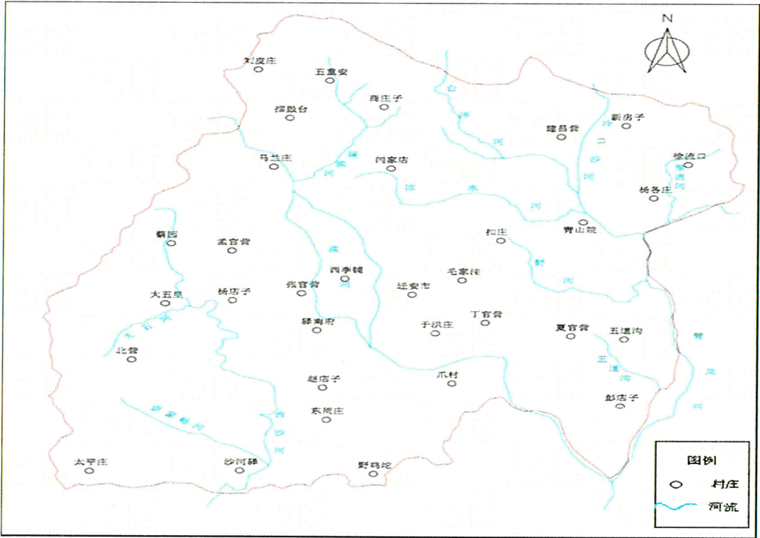
图 1- 2 迁安市水系分布图
