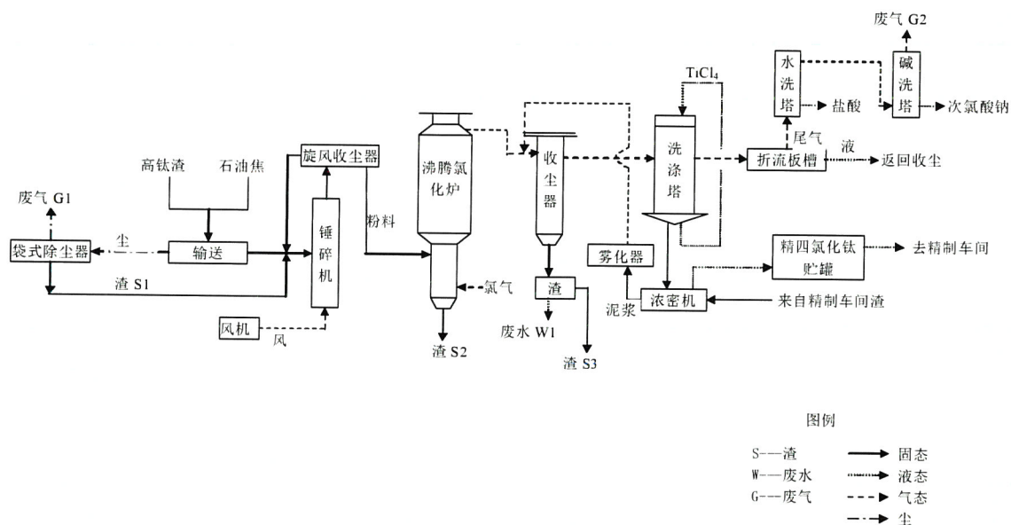
图 2-1 氯化车间生产工艺流程与排污节点图
