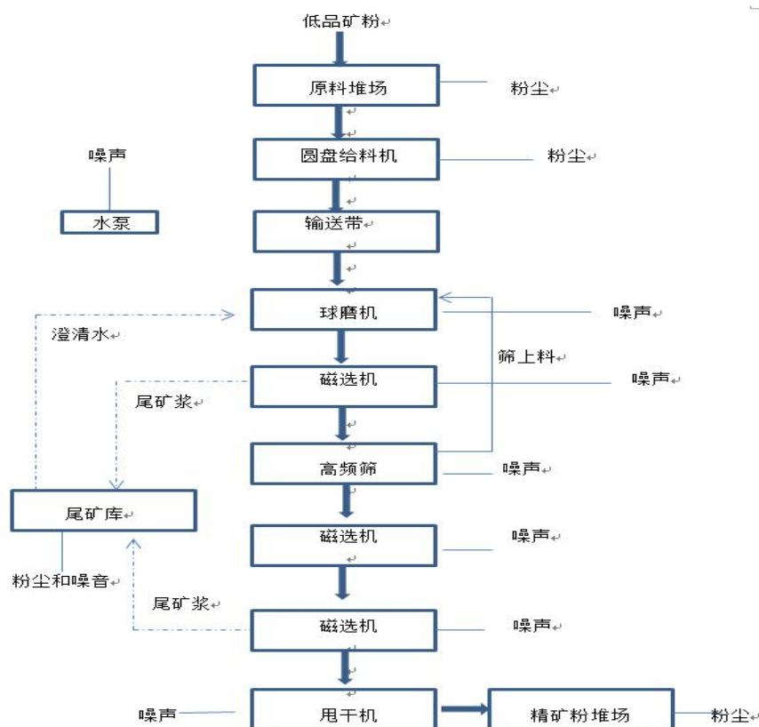
图 2-1 生产工艺流程图
