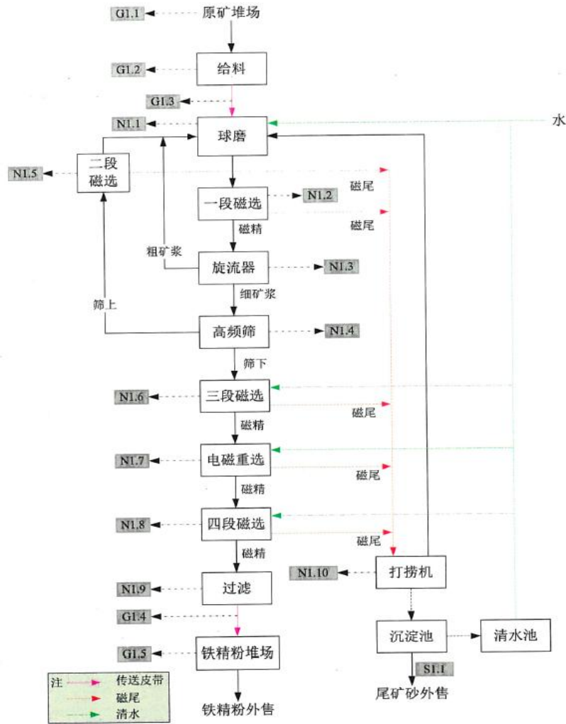
图 2-1 生产工艺流程图
